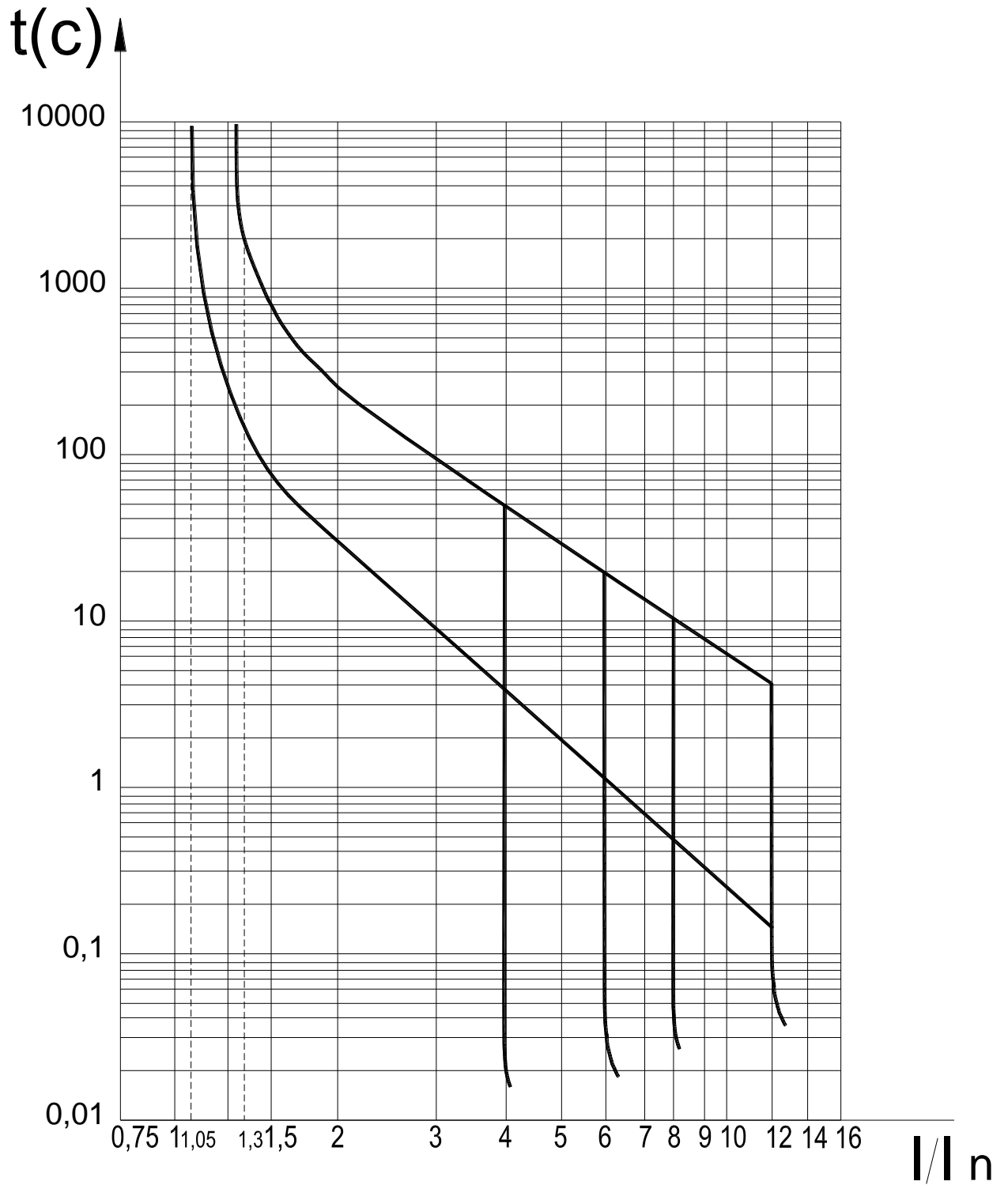
Рис. В.2 Выключатели с электромагнитными и тепловыми расцепителями с уставкой по току срабатывания 5I_n , 10I_n при температуре 30^\circ\text{C} .
