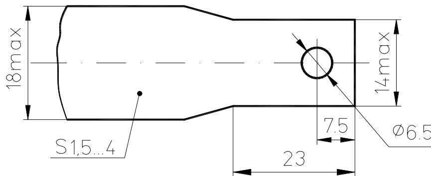
Рис.3 Форма и размеры присоединяемой шины
