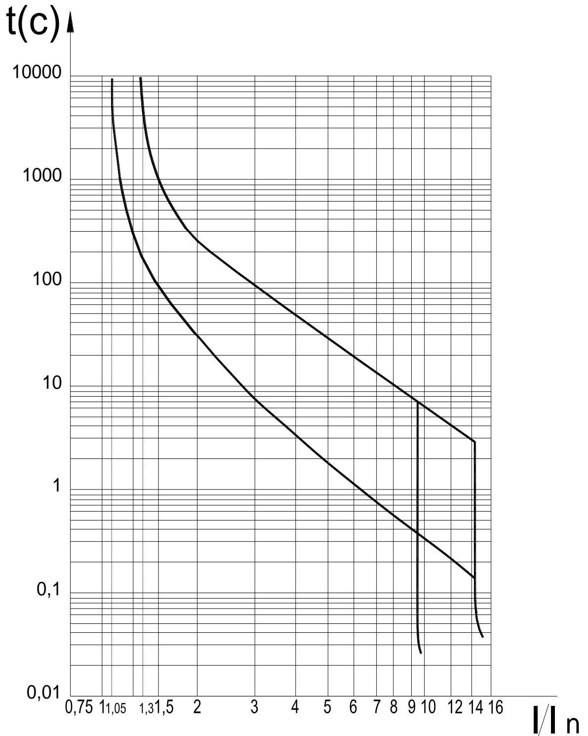
Рис. В.1 Выключатели с электромагнитными и тепловыми расцепителями с уставкой по току срабатывания 12I_n при температуре 30^\circ\text{C} .
